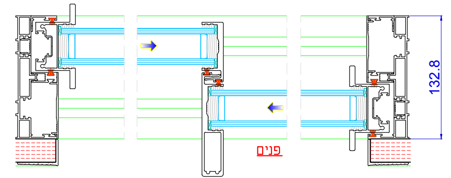
חתך A-A דו-כנפית
