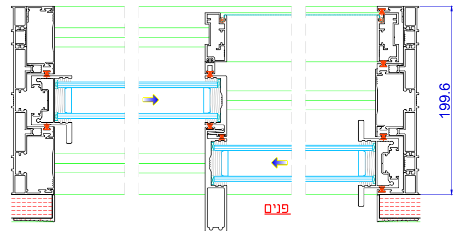
חתך C-C דו-כנפית + רשת הזזה
