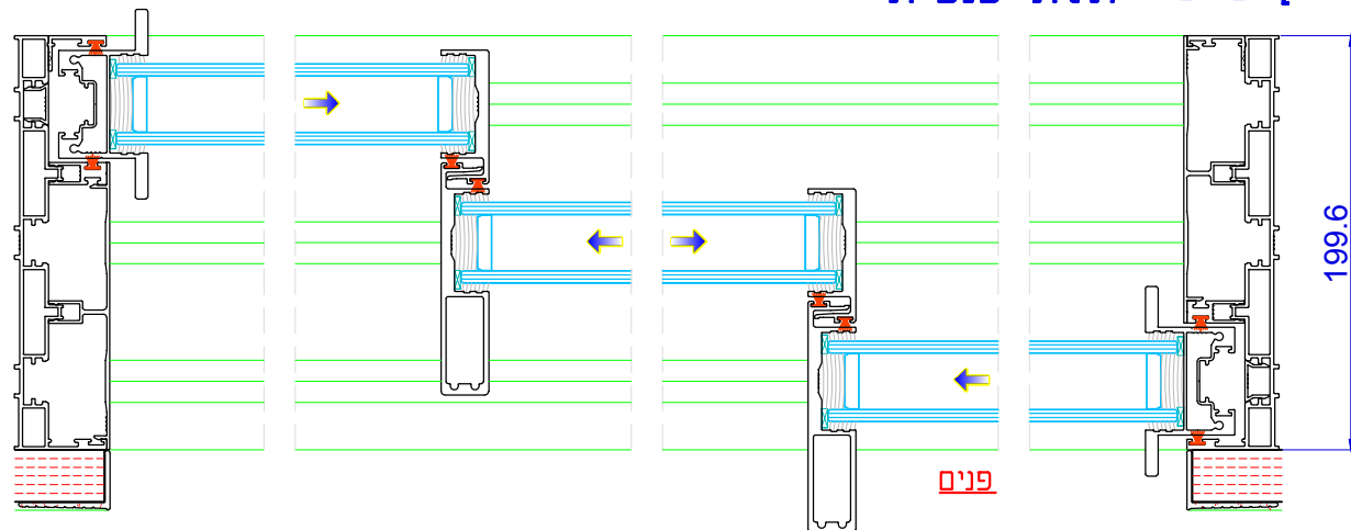
חתך D-D תלת-כנפית
