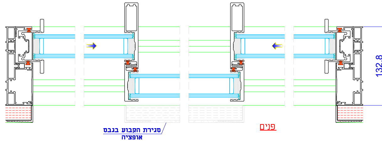
חתך B-B דו-כנפית + קבוע מרכזי
